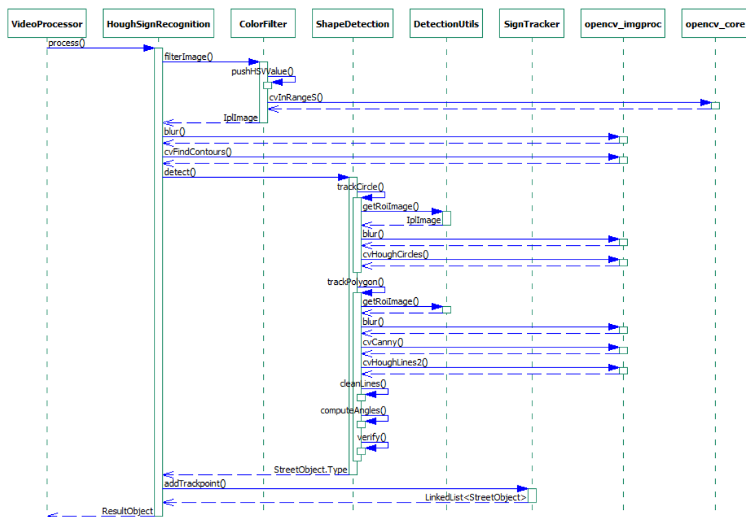
Abbildung 5-9: Das Sequenzdiagramm zeigt den Ablauf der wichtigsten Methodenaufrufe bei der Straßenschilderkennung mit dem Plugin HoughSignRecognition.
