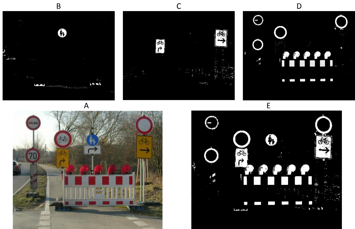
Abbildung 3-13: Bild A [31] ist das ungefilterte Originalbild. In Bild B wird ein Blaufilter verwendet, in Bild C ein Gelbfilter und in Bild D ein Rotfilter. Bild E ist das Summenbild aus B, C und D.
