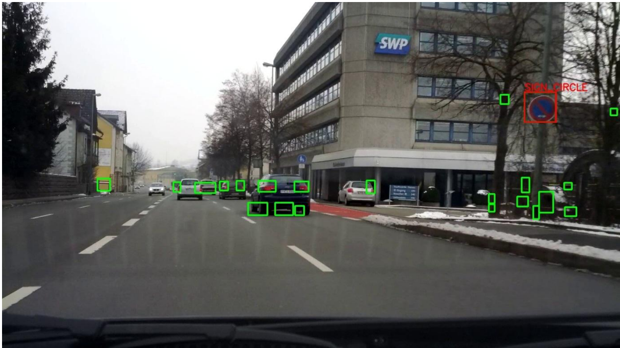
Abbildung 6-8: Erkennung eines runden Verkehrsschildes bei dunklem Hintergrund. Hier wurde kein Blaufilter gesetzt, darum ist das blaue Schild nicht als Blob gekennzeichnet.
