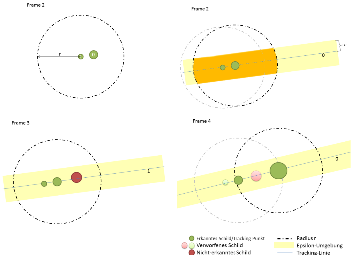
Abbildung 3-23: Grafische Darstellung des Schildverfolgungs-Algorithmus.
