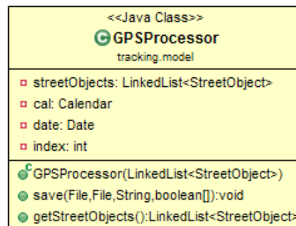
Abbildung 5-5: Die Klasse GPSPProcessor.
