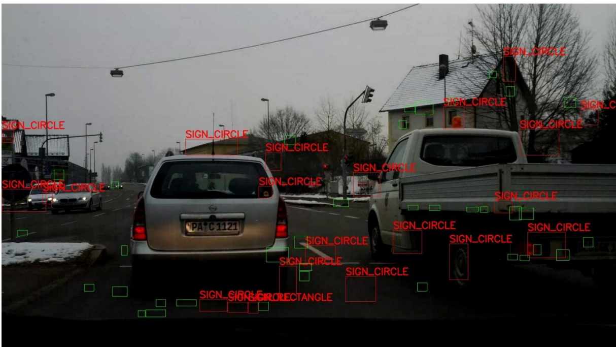
Abbildung 6-15: Durch das Setzen von sehr niedrigen Schwellwerten in der Kreiserkennung wurden Falscherkennungen provoziert.
