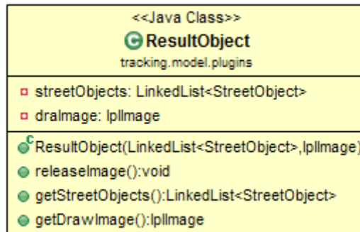
Abbildung 5-3: Die Klasse ResultObject.
