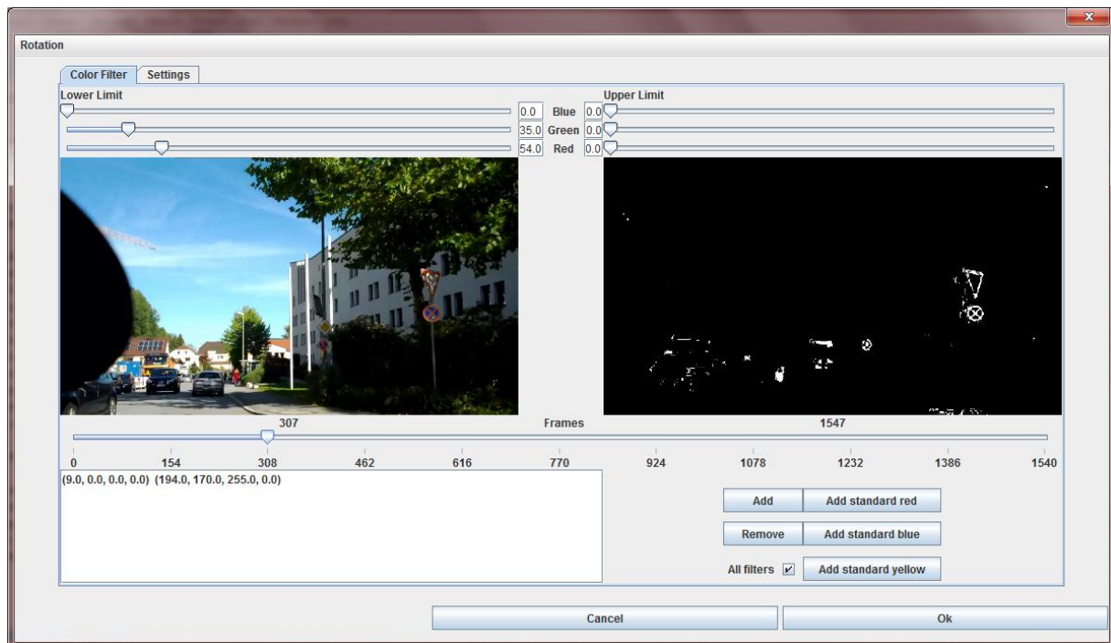
Abbildung 6-3: Einstellungsfenster für den Color Filter des Plugins HoughSignRecognition.
