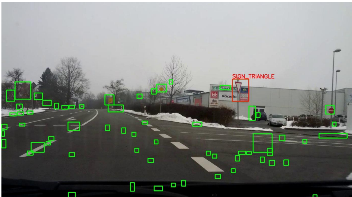
Abbildung 6-13: Erkennung eines schräg stehenden, dreieckigen Schildes. Das viereckige und das runde Schild wurden (noch) nicht erkannt.
