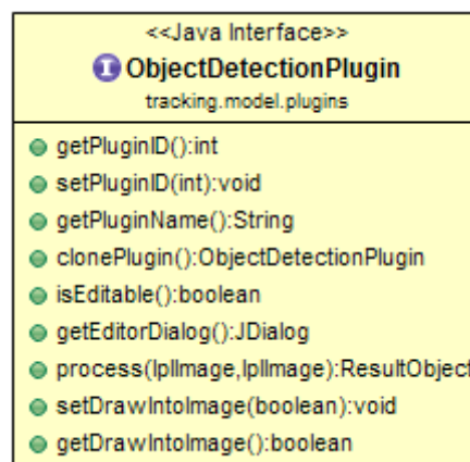
Abbildung 5-6: Das Interface ObjectDetectionPlugin .
