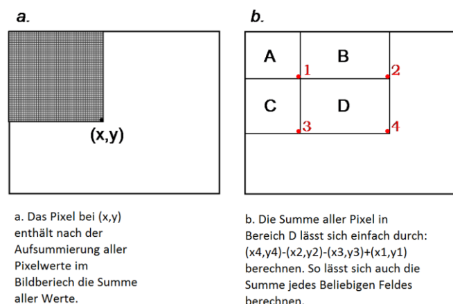
Abbildung 3-2: Funktionsweise eines Integralbilds (Integral Image). [15]
