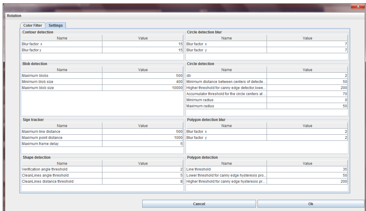
Abbildung 6-4: Einstellungsfenster für alle Parameter der Schilderkennung des Plugins HoughSignRecognition.
