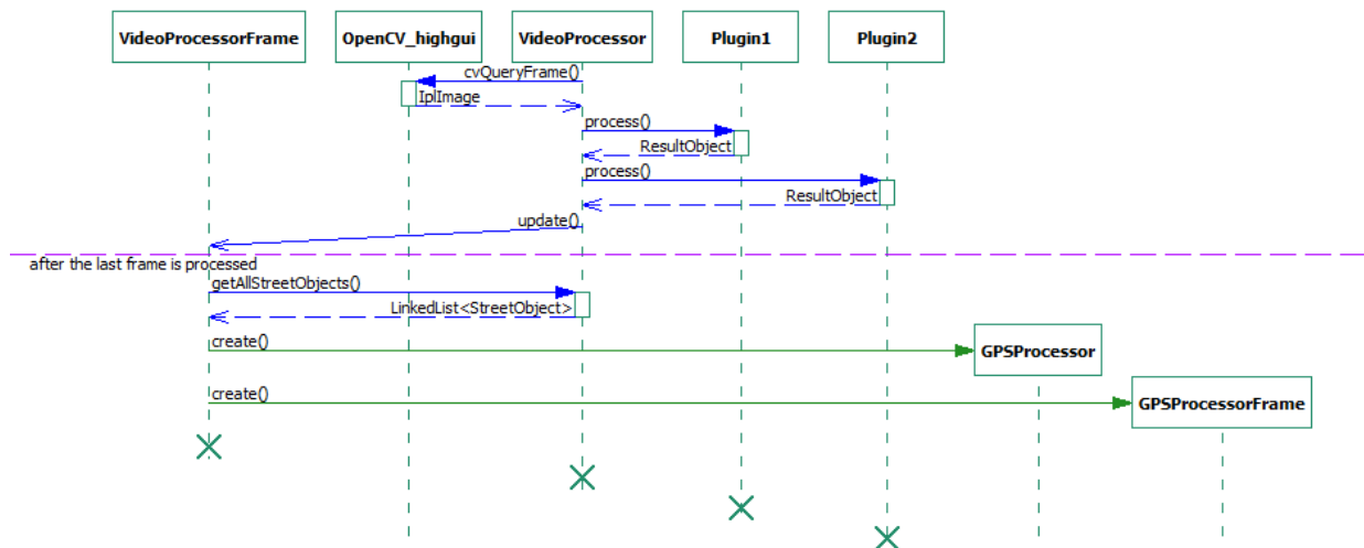
Abbildung 5-4: Das Sequenzdiagramm stellt das Einlesen und Verarbeiten der Video-Frames dar.
