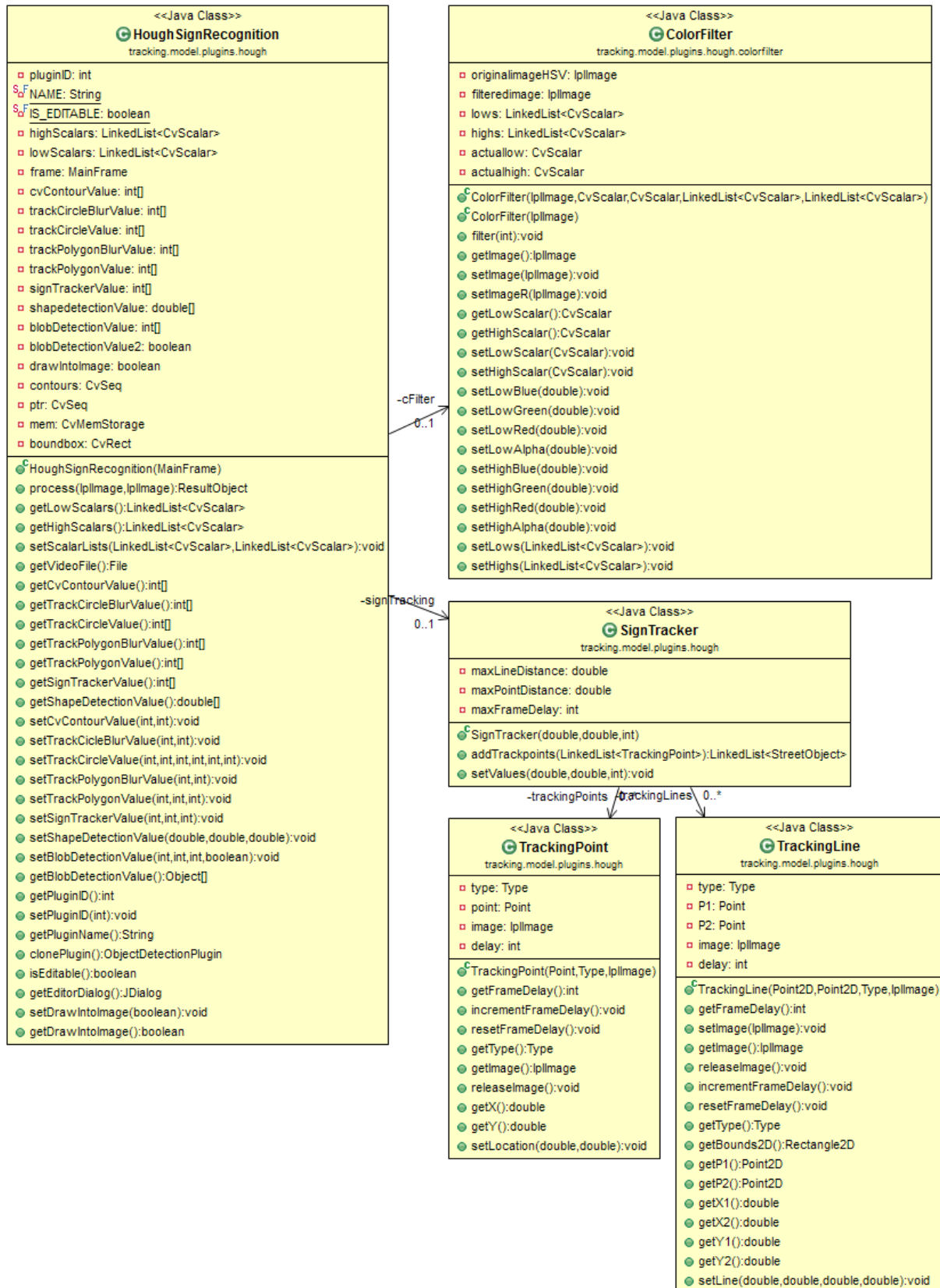
Abbildung 5-7: Hauptklassen des Plugins HoughSignRecognition.
