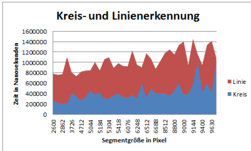
Abbildung 6-16: Verarbeitungszeiten der Kreis- und Polygonerkennung des Plugins HoughSignRecognition .
