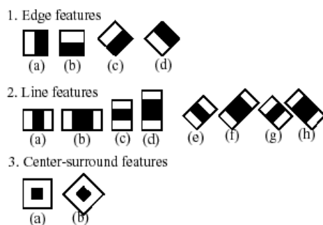
Abbildung 3-1: Einige für die Feature Detection benutzte Features. [14]
