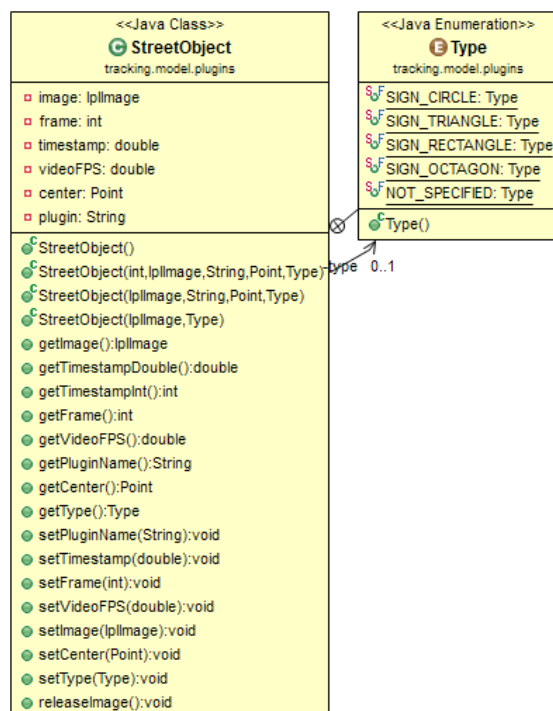
Abbildung 5-2: Die Klasse StreetObject.
