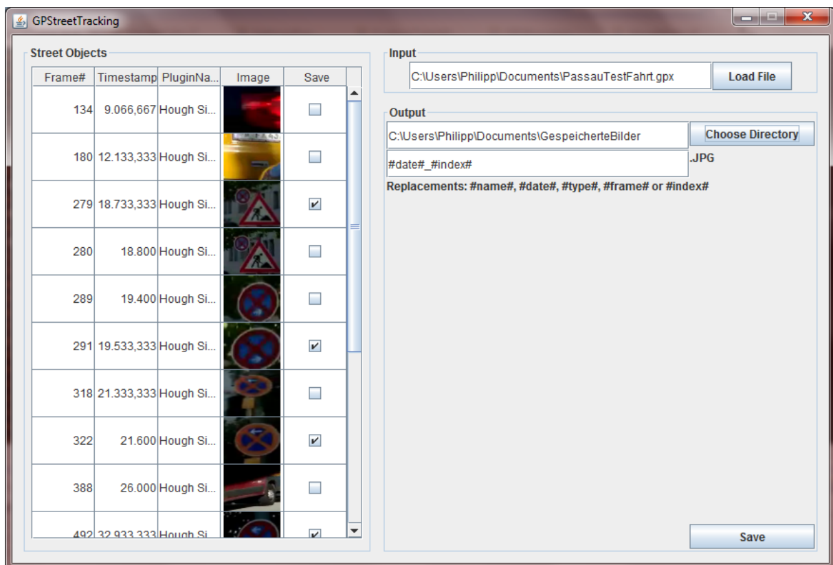
Abbildung 6-6: Objektverwaltungs- und Speicherfenster des Programms GPStreetTracker.
