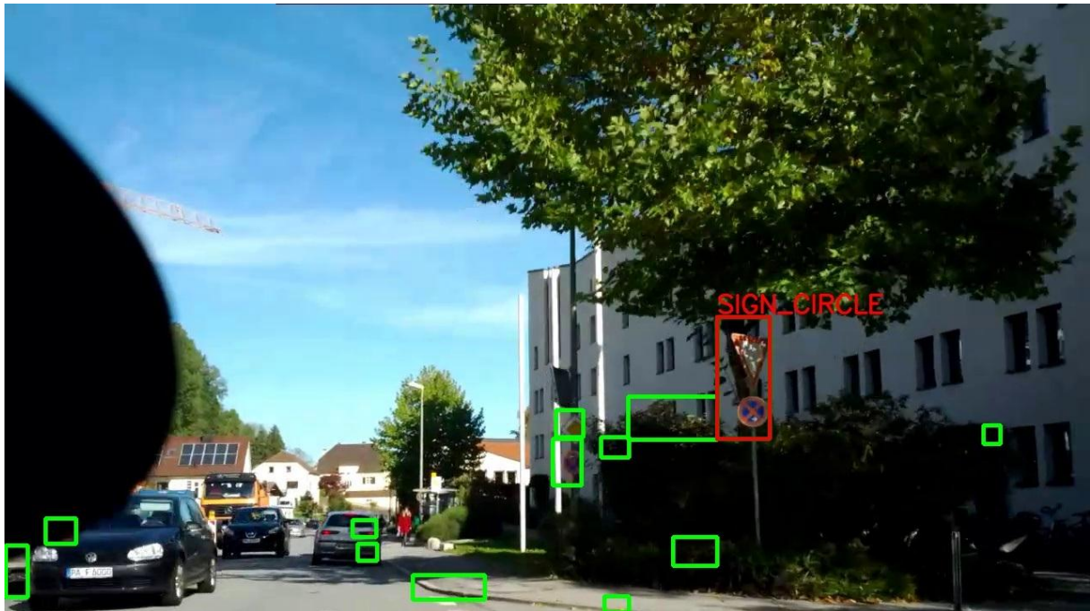
Abbildung 6-10: Erkennung eines runden Verkehrsschildes im Schatten, das dreieckige Schild wurde im selben Blob erfasst und wäre ansonsten, aufgrund der starken Lichtunterschiede auf dem Schild, nicht erkannt worden. Die beiden weiter entfernten Schilder wurden noch nicht erkannt.
