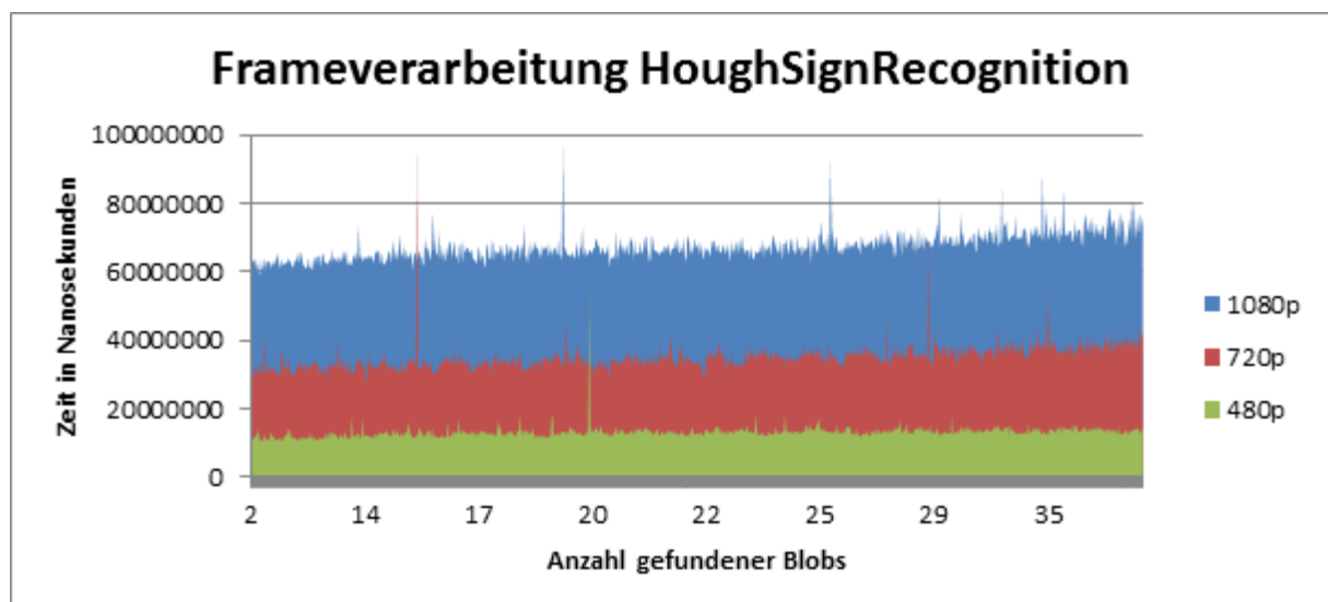
Abbildung 6-18: Verarbeitungszeit eines kompletten Frames im Plugin HoughSignRecognition .
