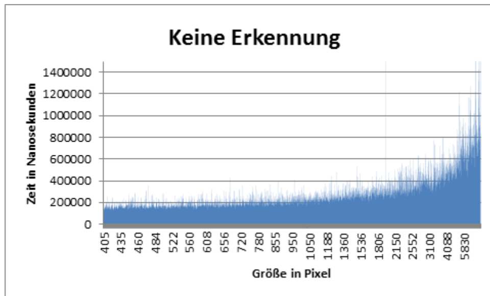
Abbildung 6-17: Verarbeitungszeiten von Bildsegmenten, in denen keine Form erkannt wird.
