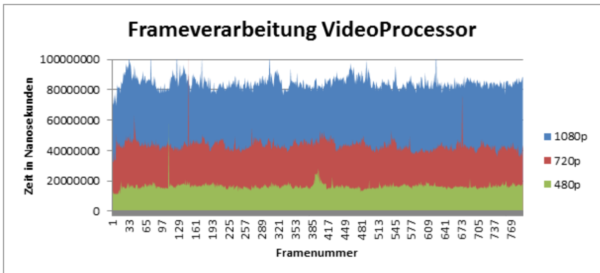
Abbildung 6-19: Verarbeitungszeit vom Einlesen eines Frames bis zum Einlesen des nächsten im VideoProcessor.
