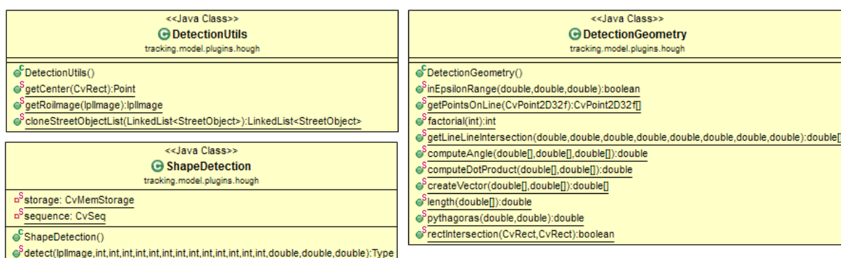
Abbildung 5-8: Statische Klassen mit Methoden zur Straßenschilderkennung.
