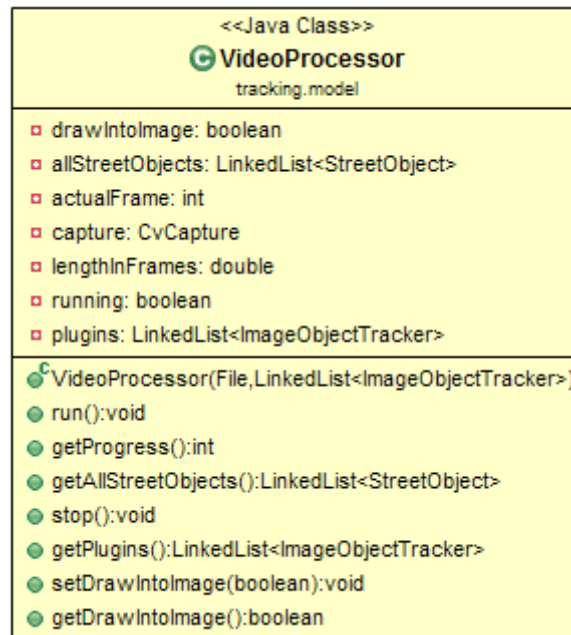
Abbildung 5-1: Die Klasse VideoProcessor.
